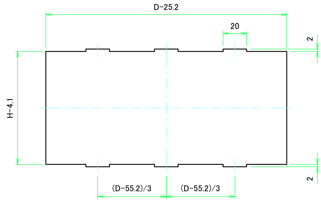
Dパネル1表面 / D Panel 1 Frontside
